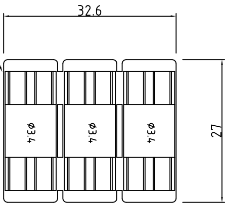
EFA04 71 P02 3.4 COUPLER CLIP
