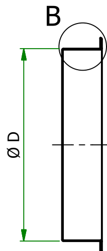
A-A ( 1 : 10 )
